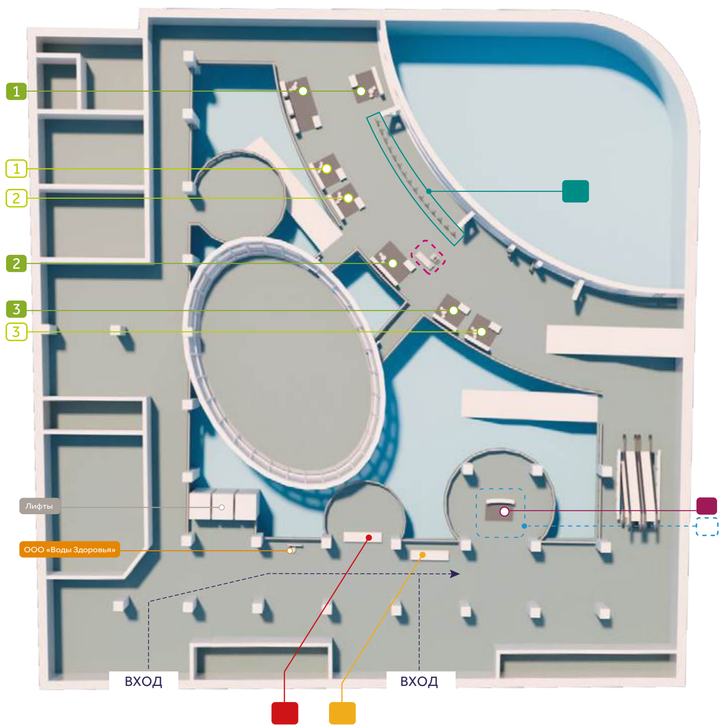
План застройки -1-й этаж
